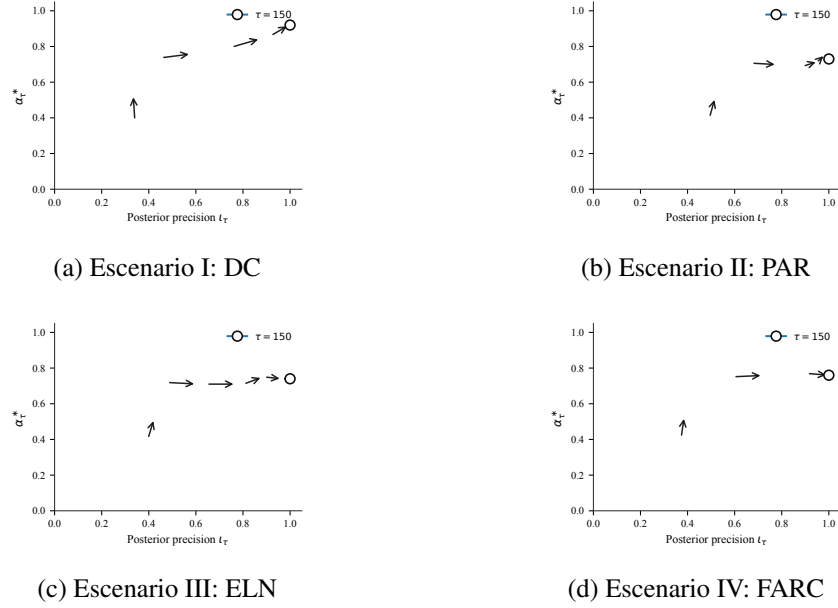
Figure IX: Trayectoria (l_t, \alpha_t^*) con flechas que indican el avance temporal.
