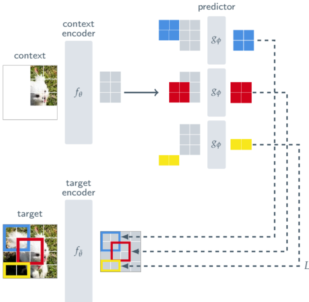
I-JEPA
