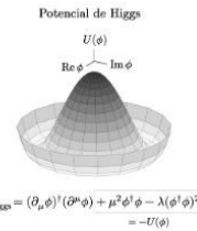
Figura 1: Representación grafica del sombrero mexicano (Potencial de Higgs).
