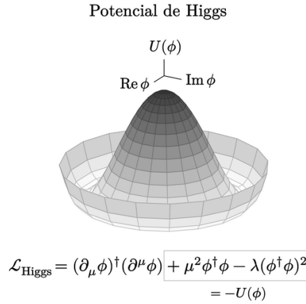
Figura 1: Representación grafica del sombrero mexicano (Potencial de Higgs).
