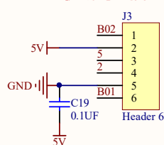
电机编码器接口2
