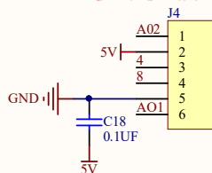
电机编码器接口1
