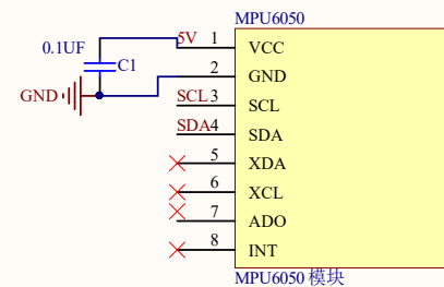
MPU6050 模块
