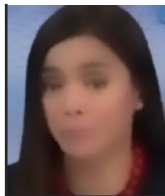
input
