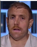
FF++ forgery
