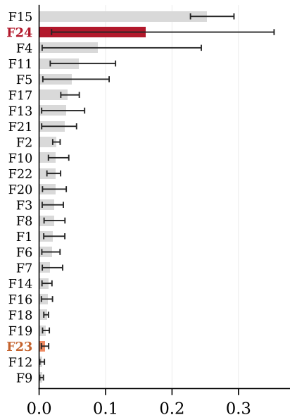
FCN
