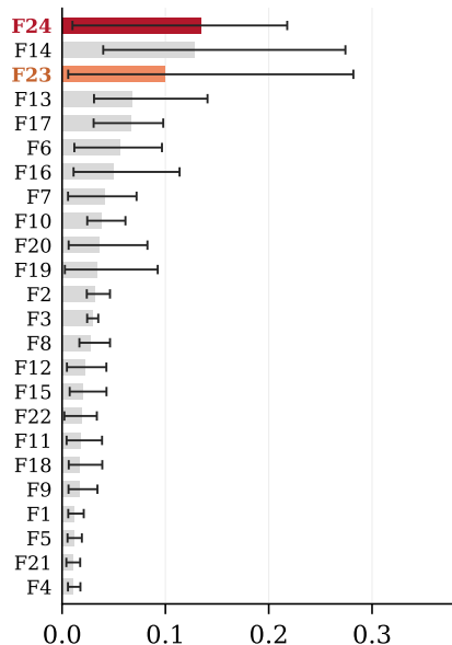
Moment
