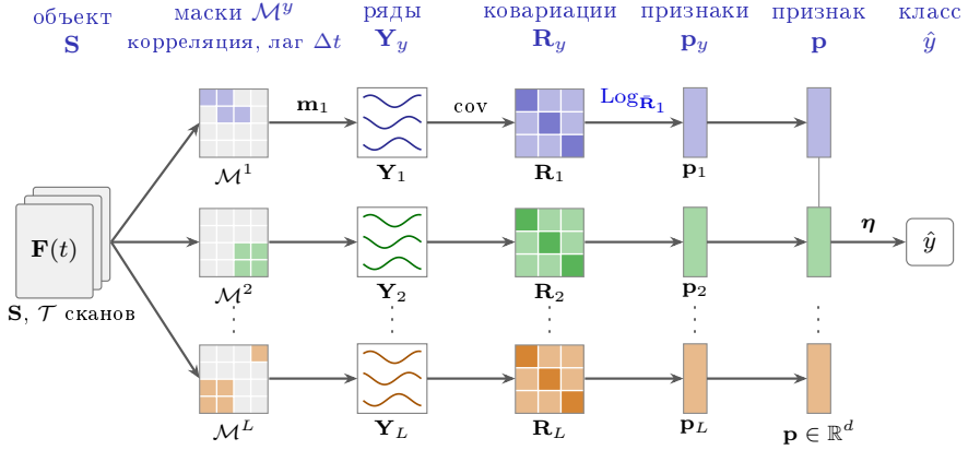
Рисунок 3 — Схема модели классификации. Маска активности M^y класса y отбирает ряды активных вокселей Y_y , их ковариационная матрица R_y проецируется на касательное пространство в точке риманова среднего \bar{R}_y , что дает вектор p_y соответствия объекта классу; векторы всех классов конкатенируются в признак p
