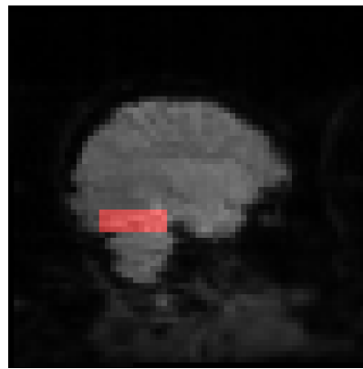
б) Алгоритм 1
