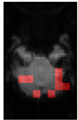
в) Алгоритм 1
