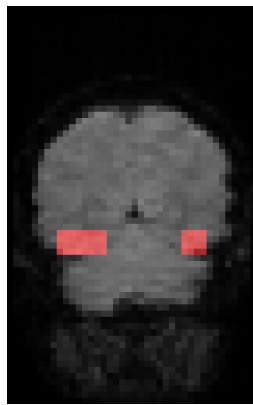
а) Алгоритм 1
