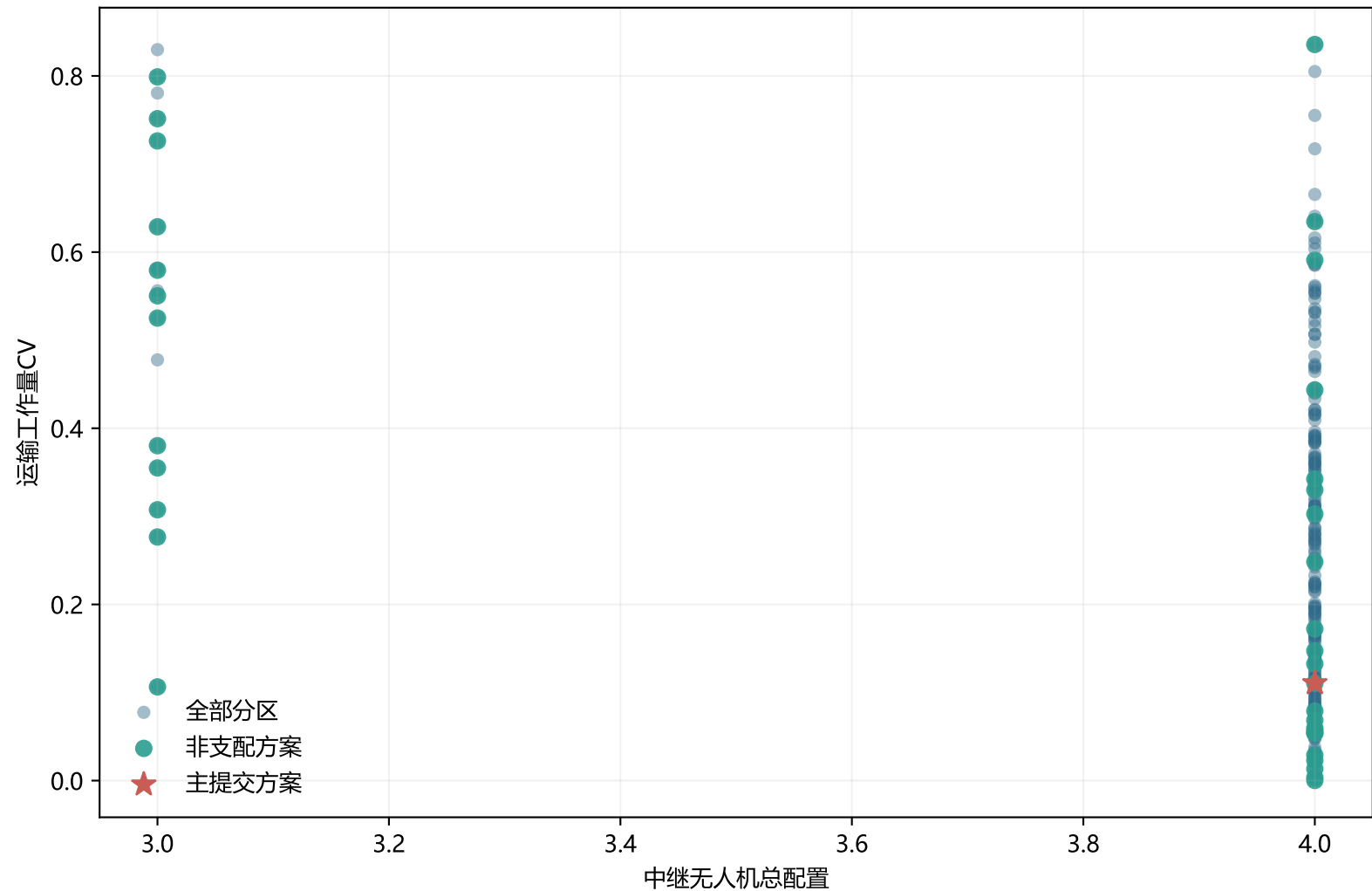
K=2 中继无人机配置—运输工作量均衡关系
