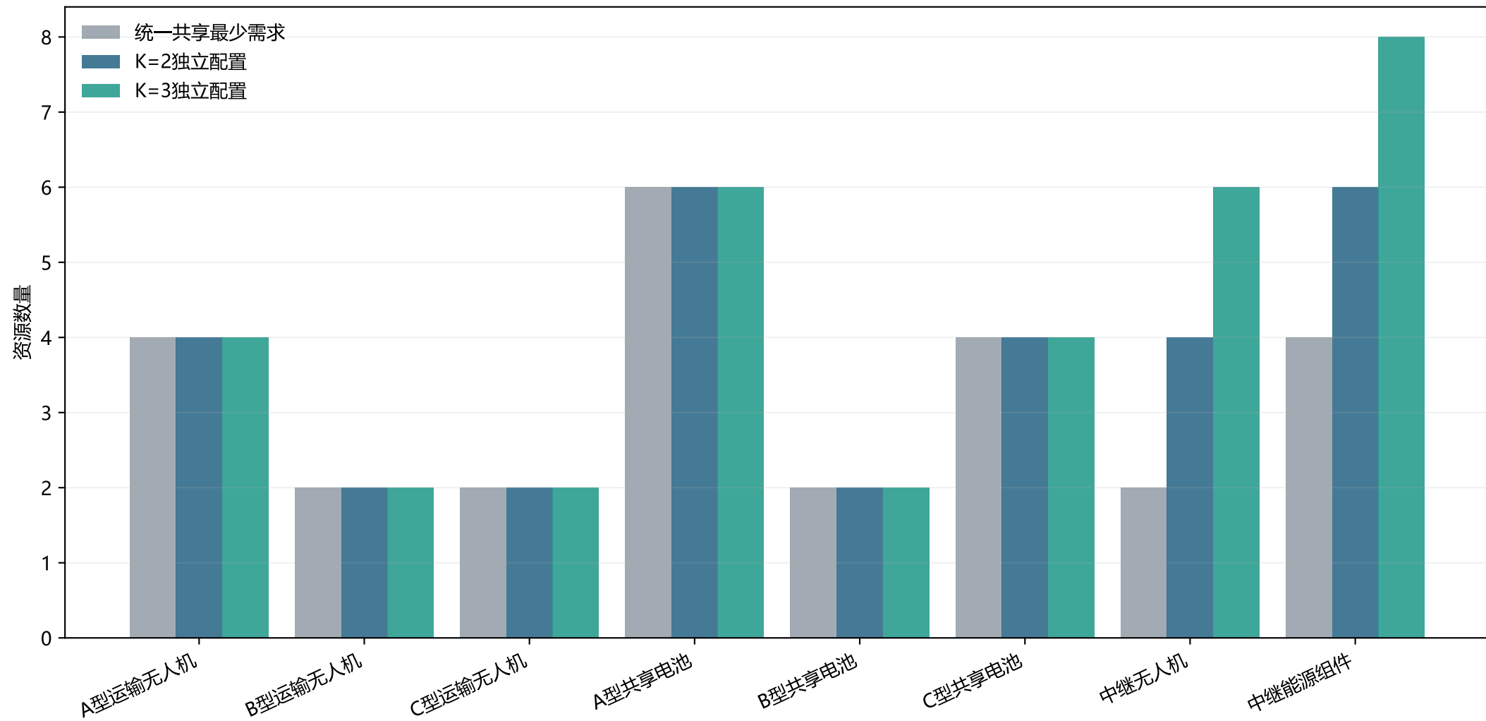
统一共享、2组独立与3组独立的资源规模比较
