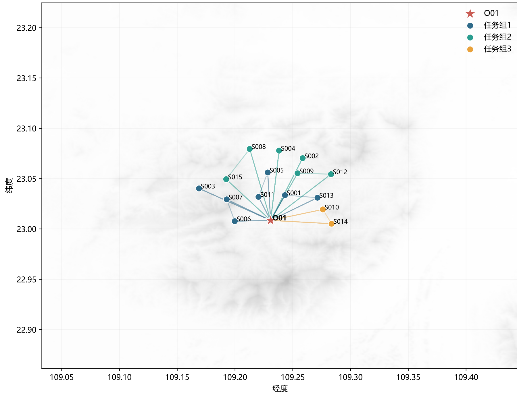
K=3 主方案固定运输路线与空间分区
