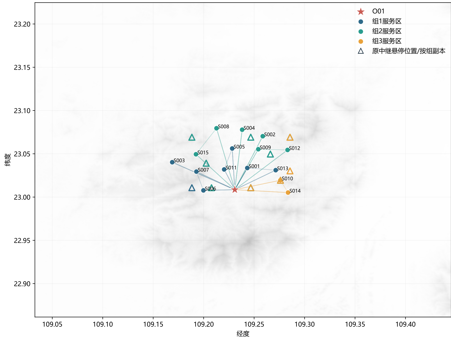
K=3 运输—分区—中继复制空间综合图
