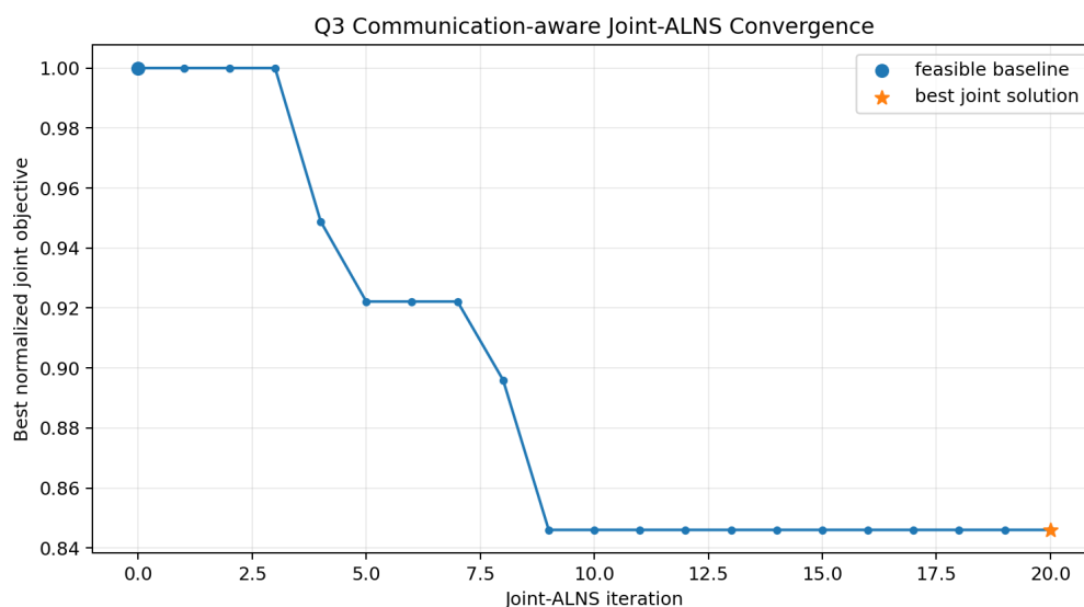
图 11 问题三通信感知 Joint-ALNS 收敛曲线
