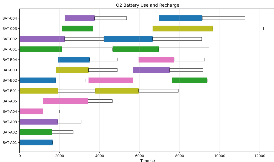
图 5 问题二共享电池使用与充电周转时序
