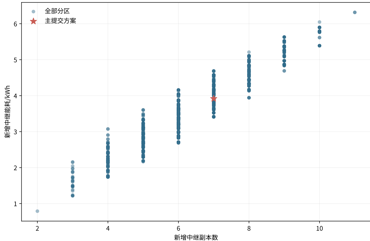
K=3 中继副本数量—新增能耗关系
