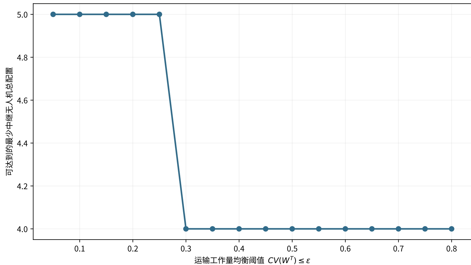
K=3 均衡要求对中继资源下界的敏感性
