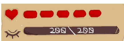
(图 5.3-2 属性 UI)
