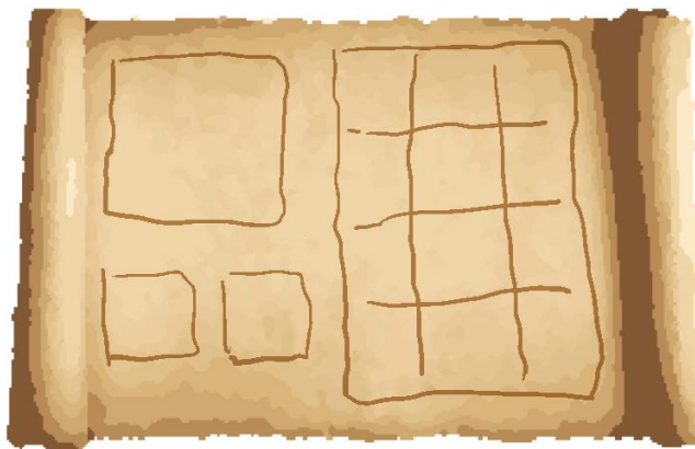
(图 5.3-1 背包界面)
