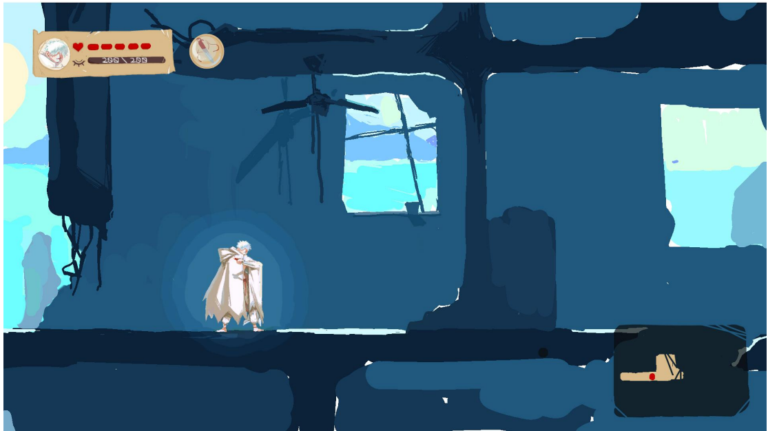
(图 5.2-1 战斗界面)
