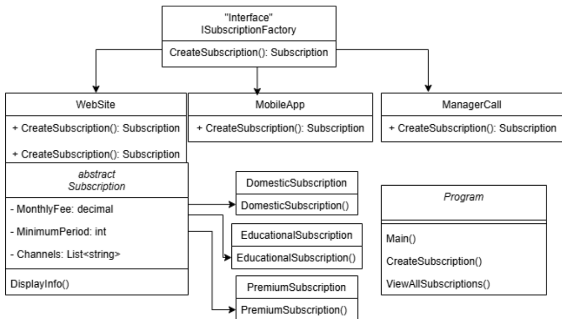
Діаграма класів:
