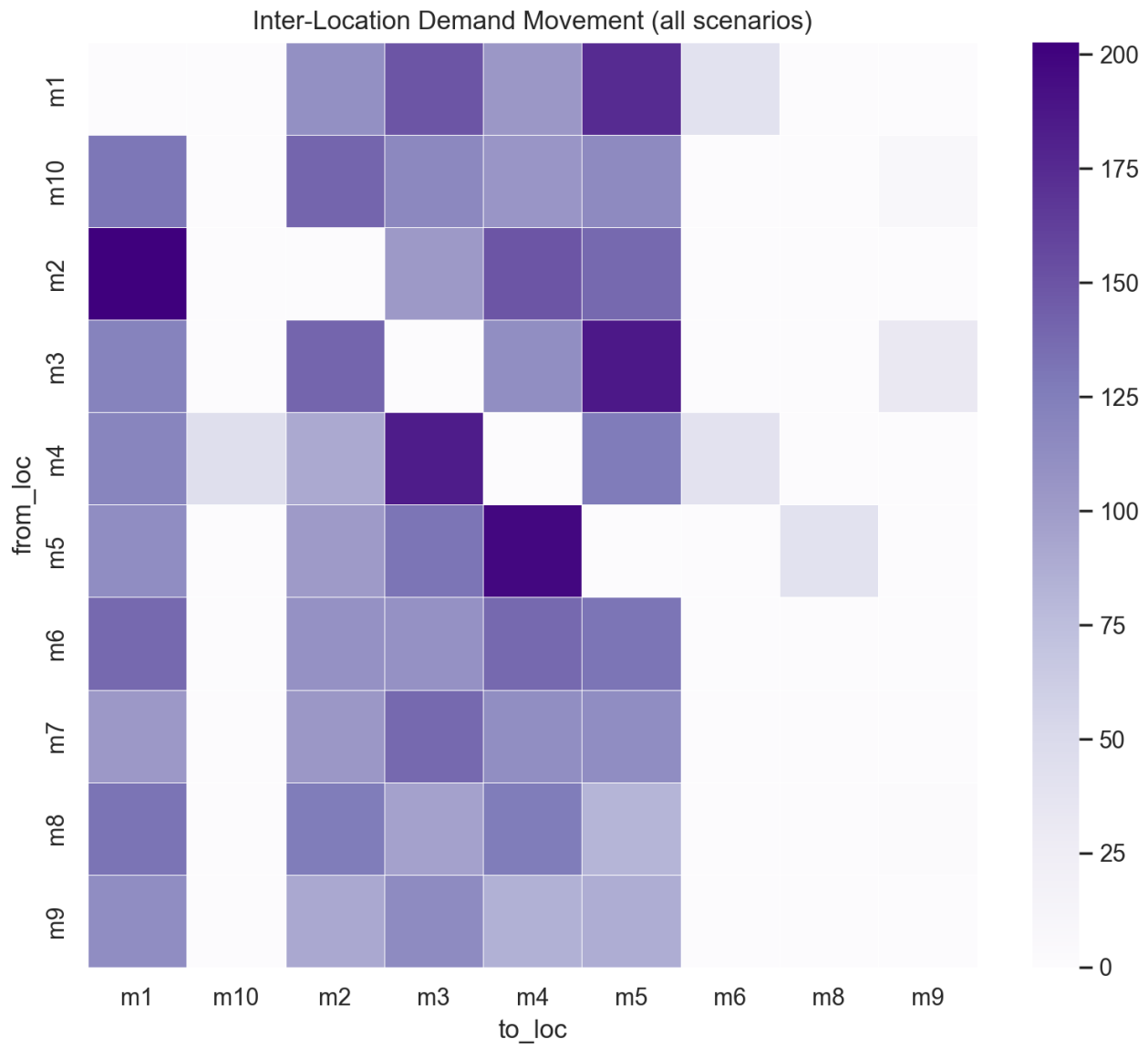
movement_heatmap_(all_scenarios).png
