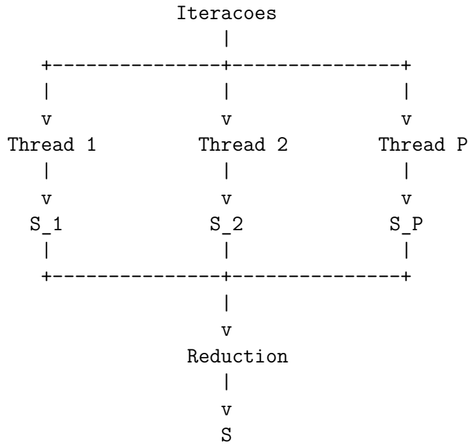
Figura 6.6: Estratégia conceitual utilizada pela redução.
