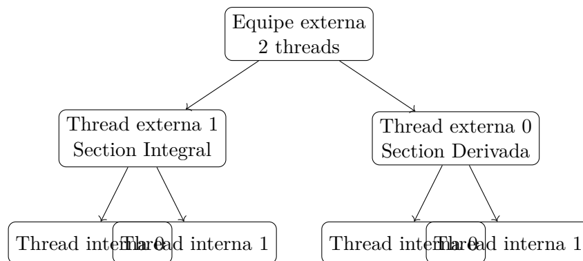
Figura 8.3: Distribuição de threads observada na execução da Atividade 8.
