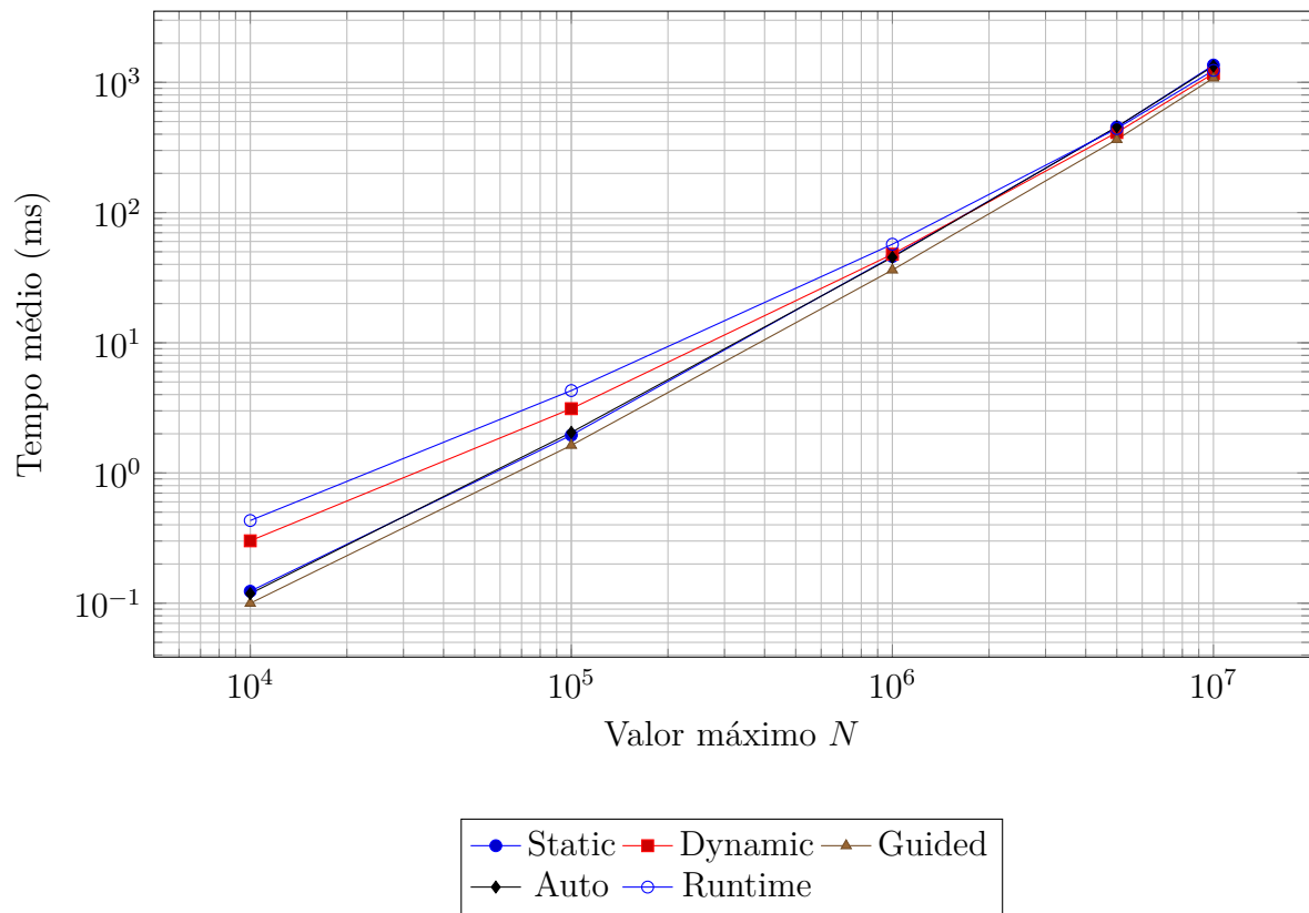
Figura 7.2: Tempo médio das políticas de escalonamento utilizando reduction .
