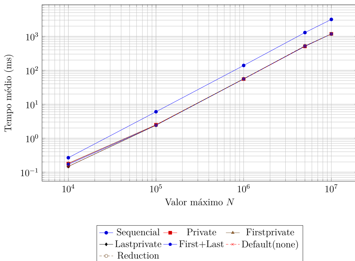
Figura 7.1: Tempo médio das versões de escopo de dados. As versões funcionalmente incorretas são exibidas apenas para caracterização experimental e não constituem soluções válidas para a contagem global.
