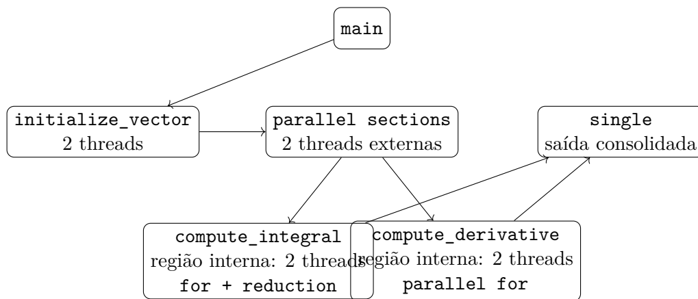
Figura 8.1: Representação estrutural da implementação da Atividade 8.
