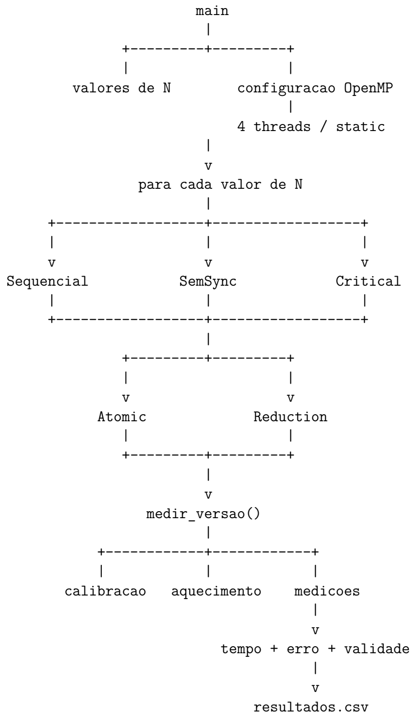
Figura 6.1: Estrutura geral da implementação da Atividade 6.
