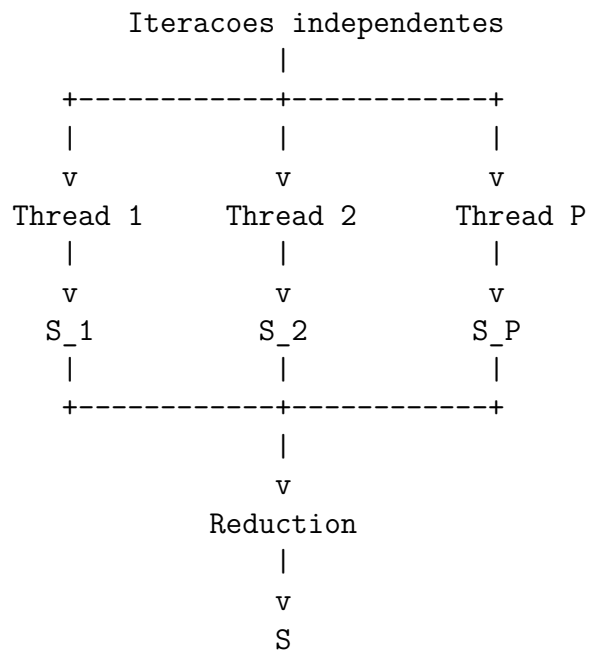
Figura 4.3: Decomposição conceitual do acumulador por redução.
