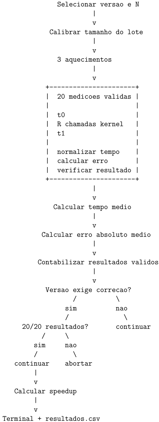
Figura 6.2: Fluxo experimental utilizado para cada implementação.
