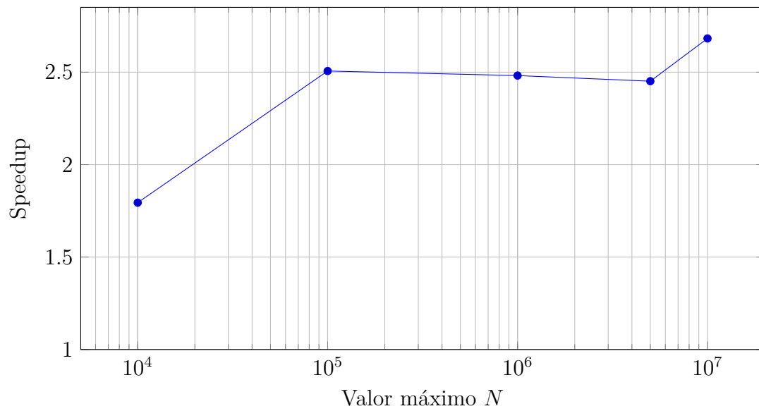
Figura 7.3: Speedup da implementação reduction + static em relação à versão sequencial no experimento de escopo de dados.
