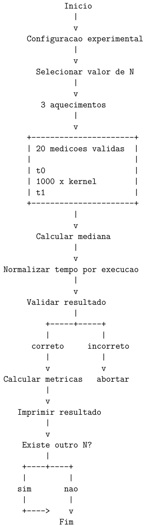
Figura 4.2: Fluxo de execução do benchmark sequencial.
