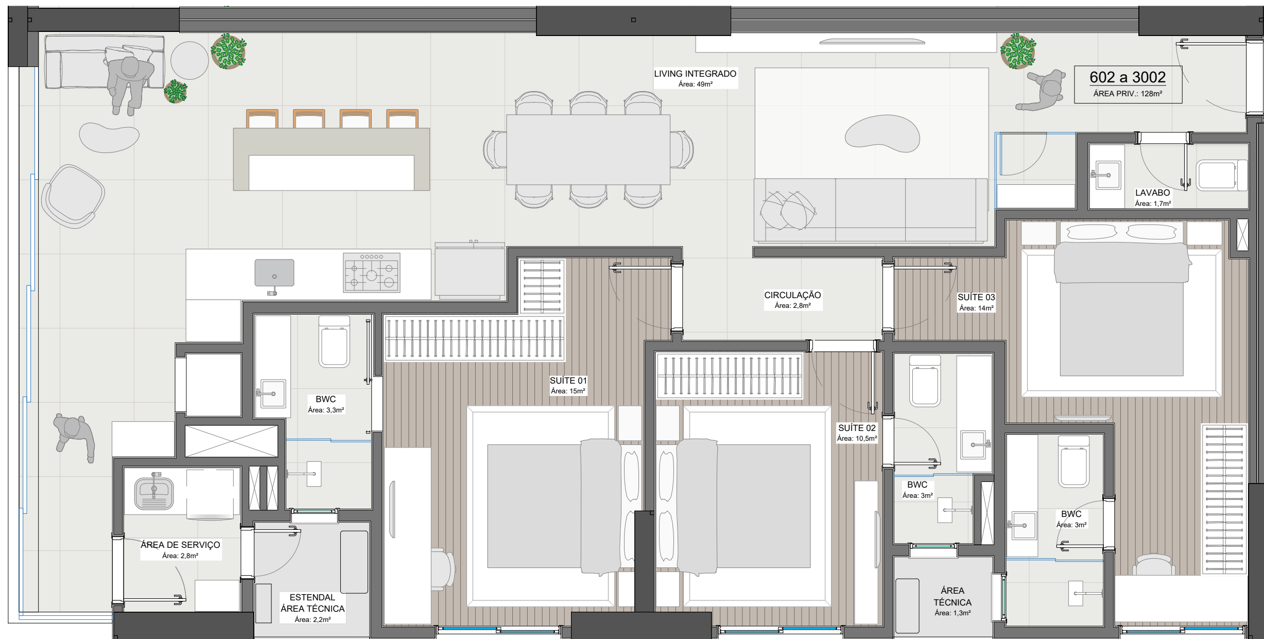
TIPO 02 ESC.: 1:50
