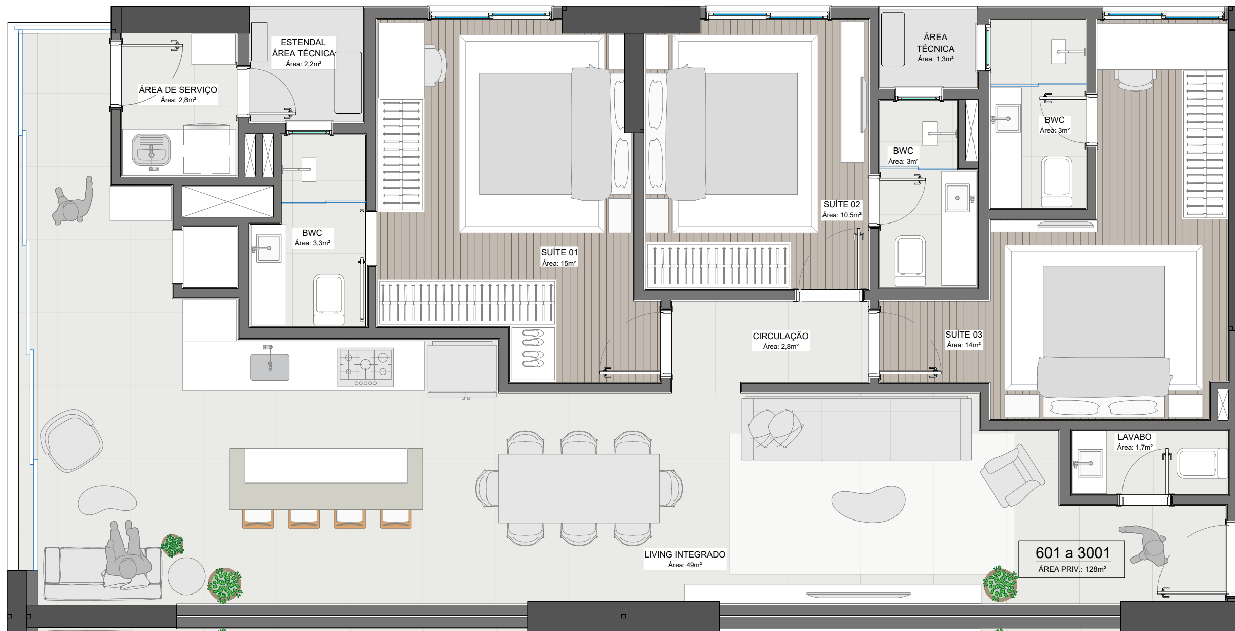
TIPO 01 ESC.: 1:50
