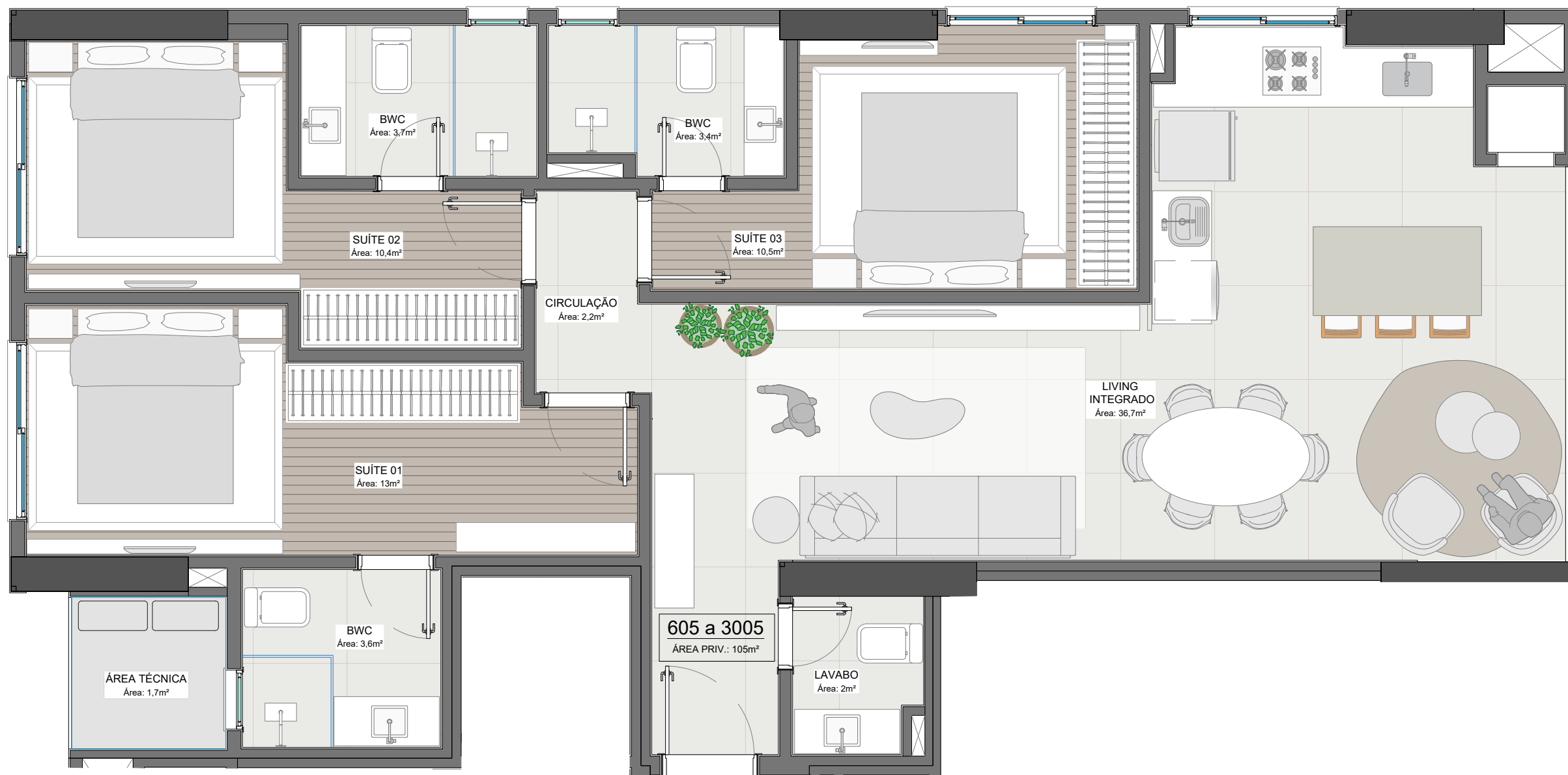
TIPO 05 ESC.: 1:50
