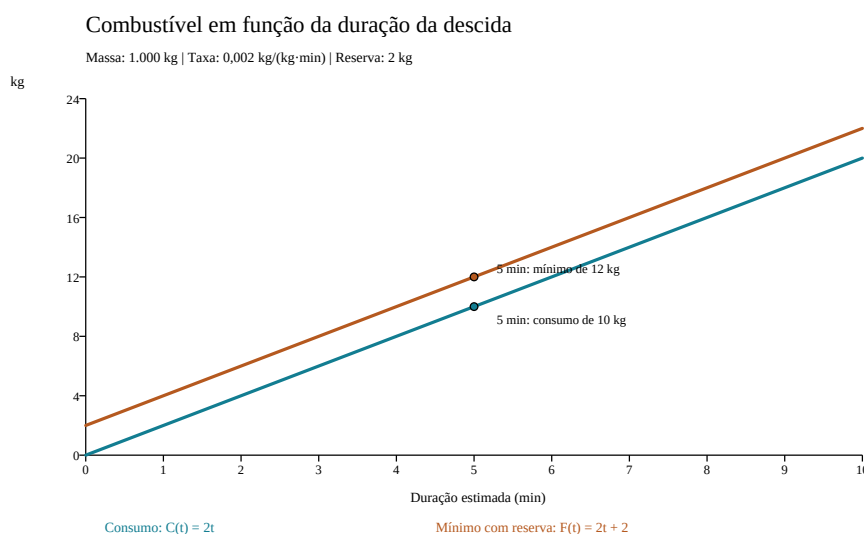
Figura 2. Consumo estimado e mínimo com reserva para massa de 1.000 kg. Elaborado a partir da fórmula e dos parâmetros do protótipo.
