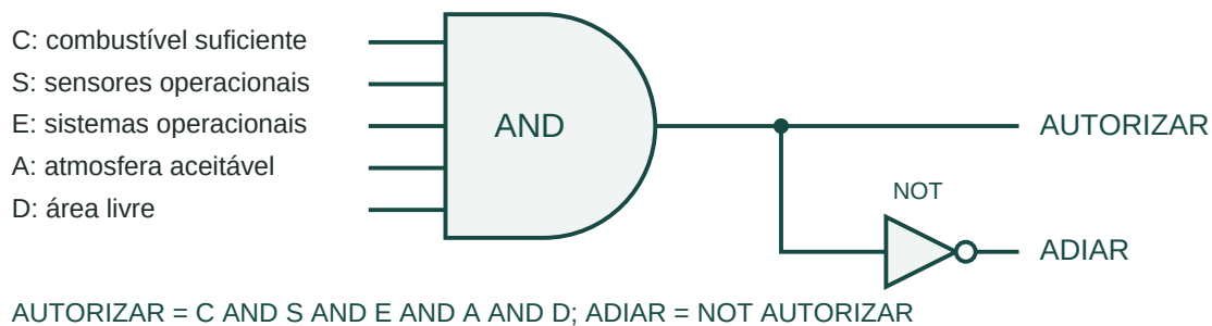
Figura 1. A porta AND reúne as condições obrigatórias. A porta NOT representa a decisão de adiar quando a autorização é falsa.
