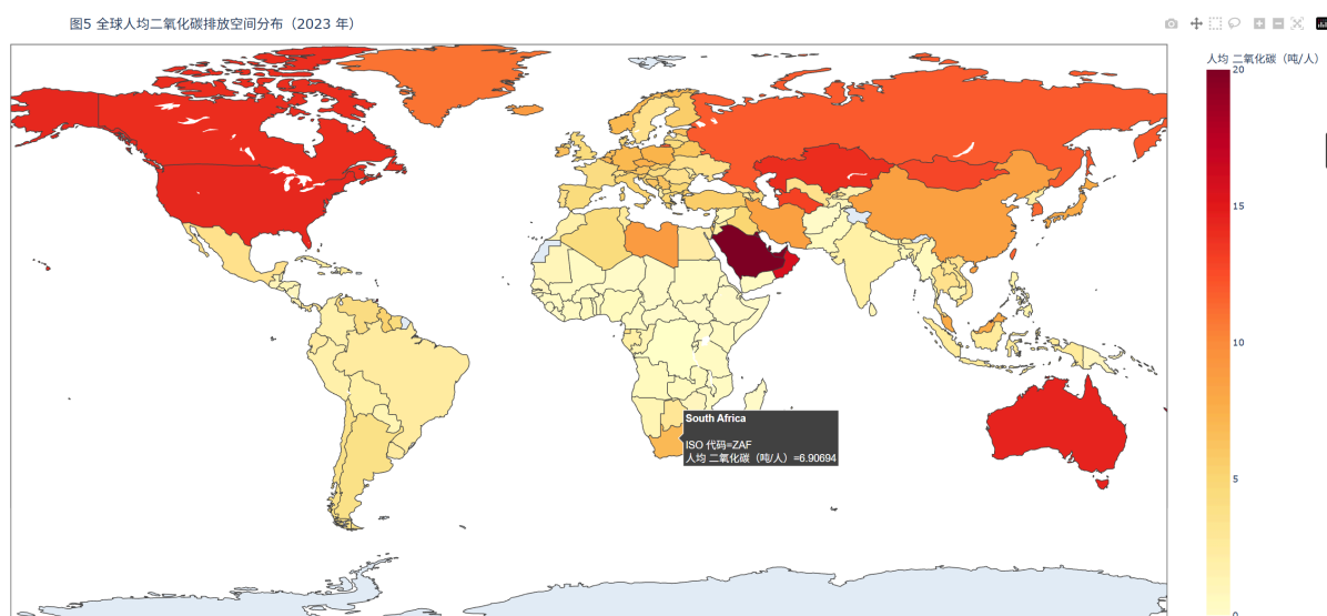
图 5 图 5 全球人均 CO 2 排放空间分布 ( 2023 年 )
