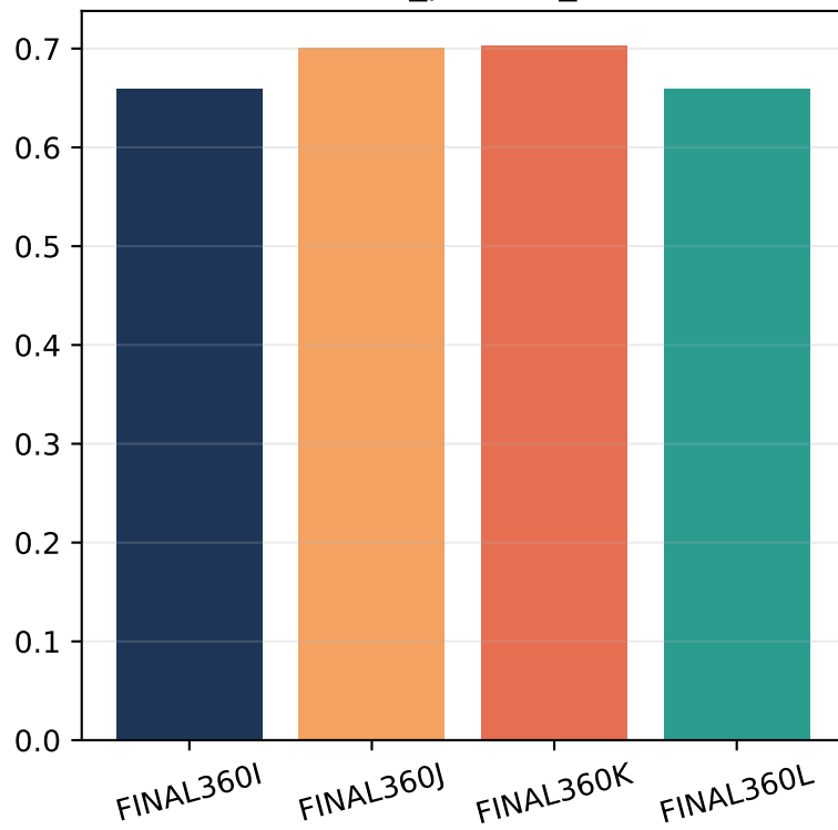
val anti_parallel_rate
