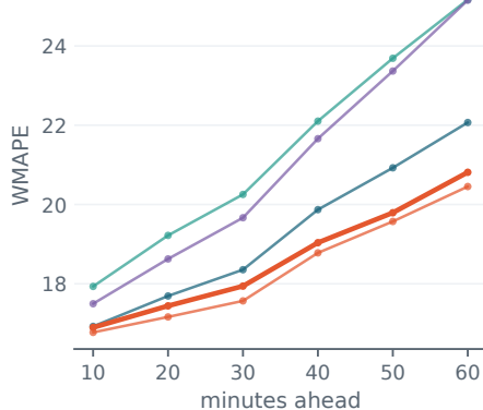
(b) WMAPE
