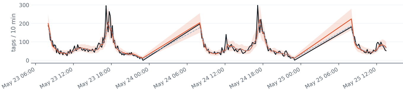
(d) Station 39 — entry, +10 min (WMAPE 19.2%)
