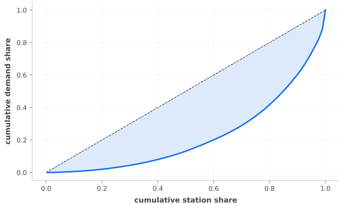
Lorenz curve (Gini=0.556)
