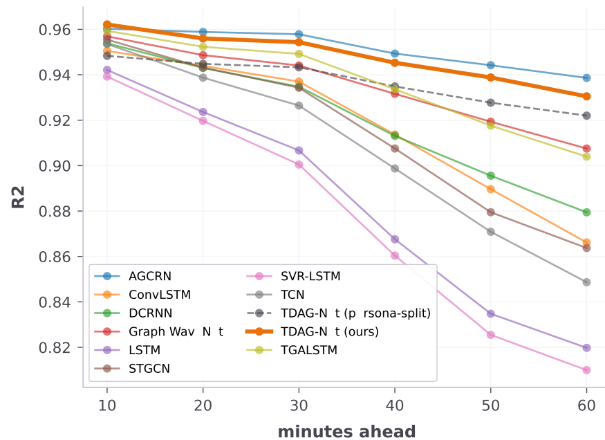
R2
