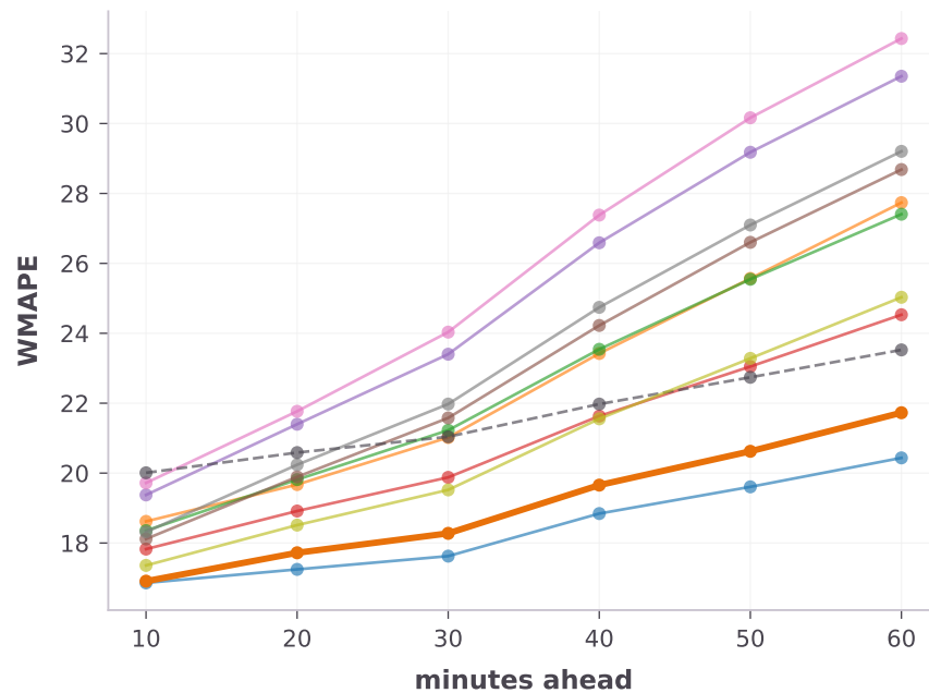
WMAPE
