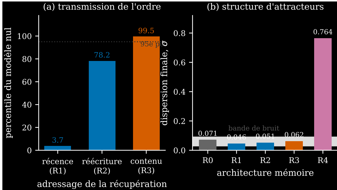
Figure 2: Transmission de l'ordre et structure d'attracteurs sont séparables. (a) La transmission de l'ordre croît de façon monotone avec l'adressage de la récupération ; seul l'adressage par contenu dépasse le modèle nul. (b) Dispersion des points d'arrivée : toute architecture naturelle, R3 comprise, demeure à l'intérieur de la bande de bruit de l'instrument ; seul l'état explicite couplé à la perception (R4, violet) produit des bassins larges.
