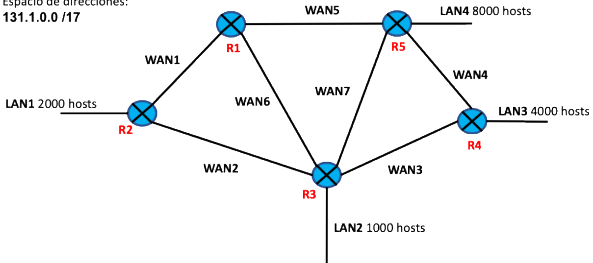
Figura 1. Topología de red de una organización.
