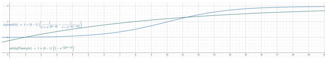
Figure 9: Vergleich der Sigmoid-Funktion und der Utility-Theory-Funktion. Die X-Achse zeigt die Anzahl positiver Detektionen abzüglich des Initialwertes ( n - 1 ), die Y-Achse den resultierenden Gewichtungsfaktor.
