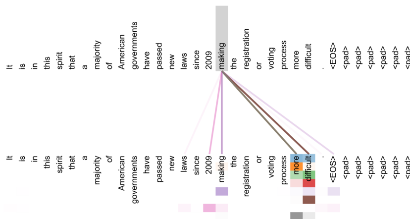
Figure 8: Visualisierung der Attention-Mechanismen (adaptiert nach Figure 3 aus [13])
