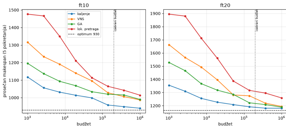
Slika 3.1: Prosečna vrednost funkcije cilja u zavisnosti od dodeljenog budžeta, za dve najteže instance. Obe ose prikazane su za pet nezavisnih pokretanja po tački. Usppravna isprekidana linija označava budžet usvojen u ostatku rada.
