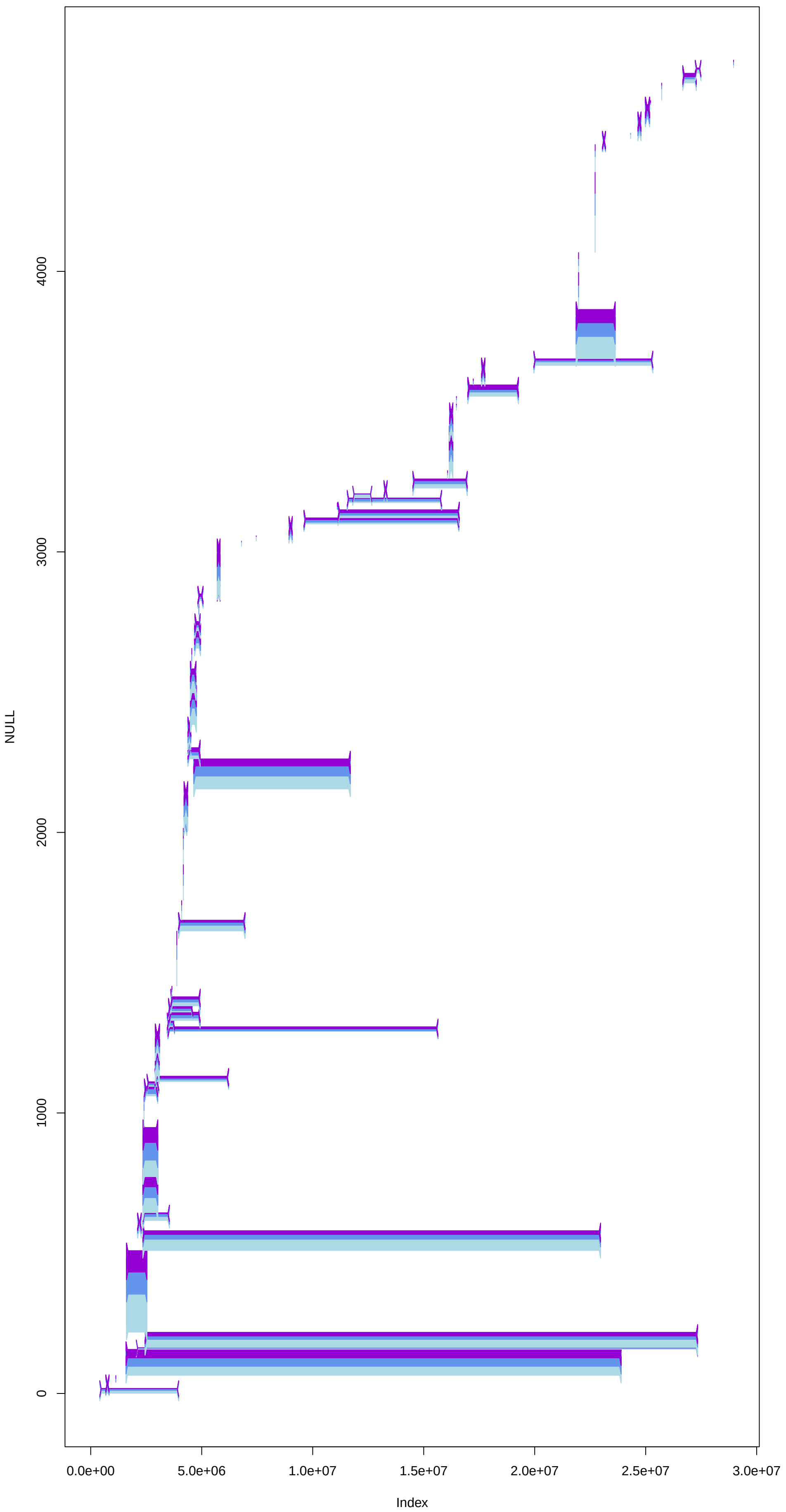
NC_044055.1
