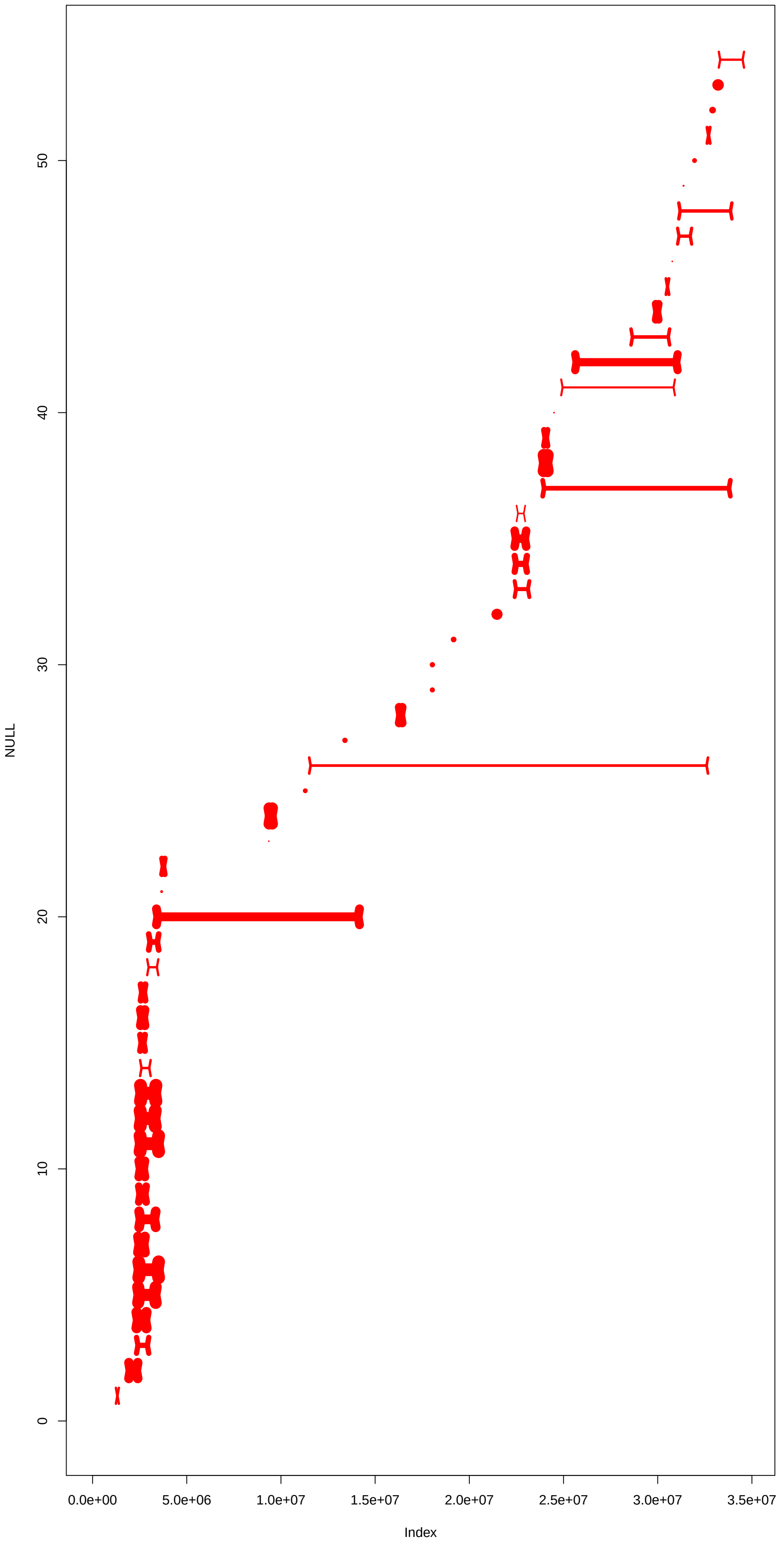
NC_044063.1 pass2
