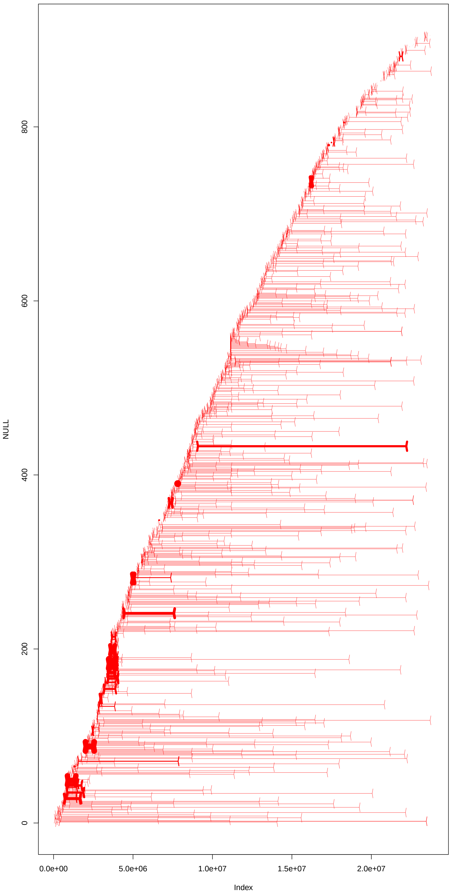
NC_044069.1
