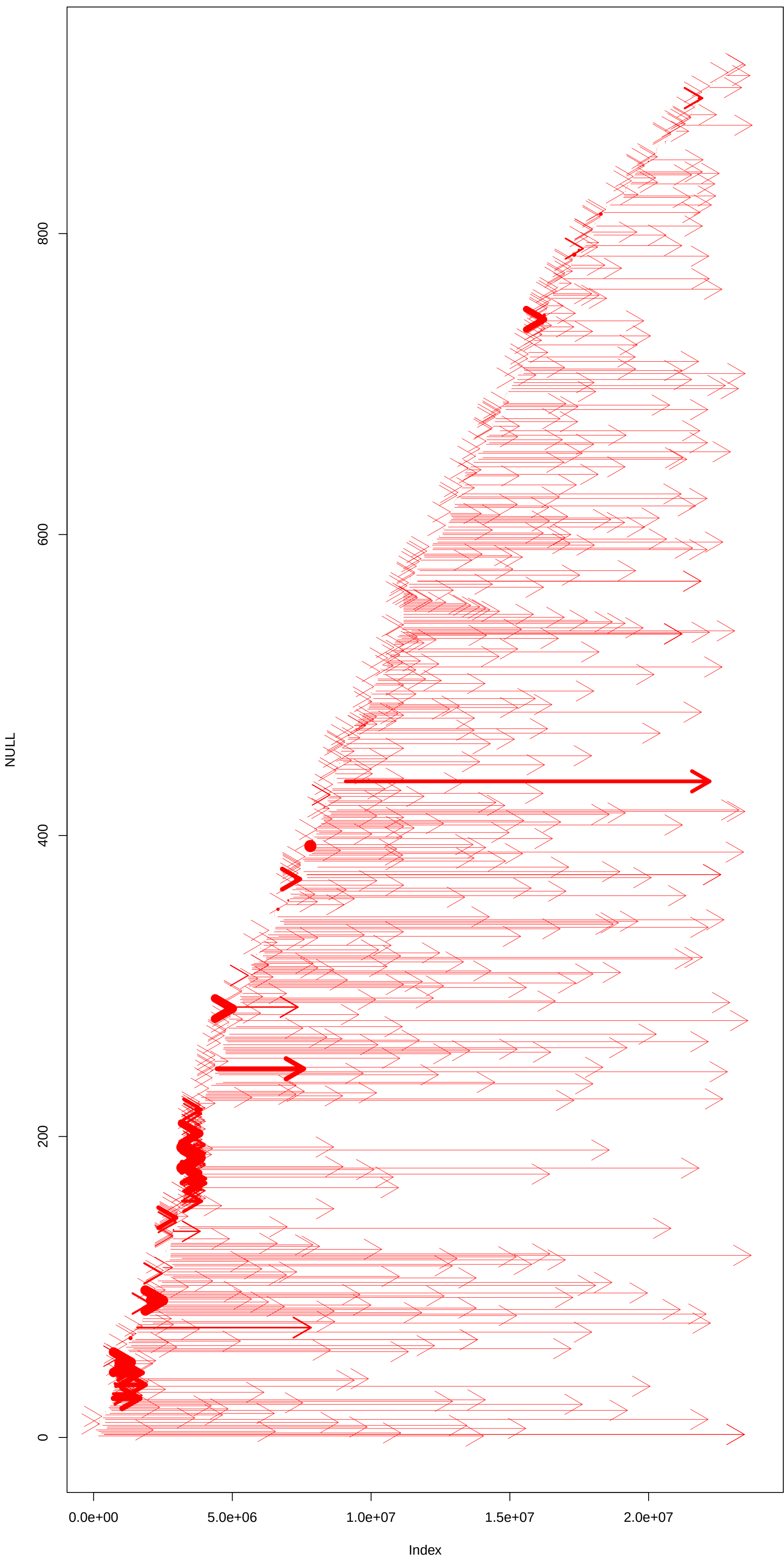
NC_044069.1
