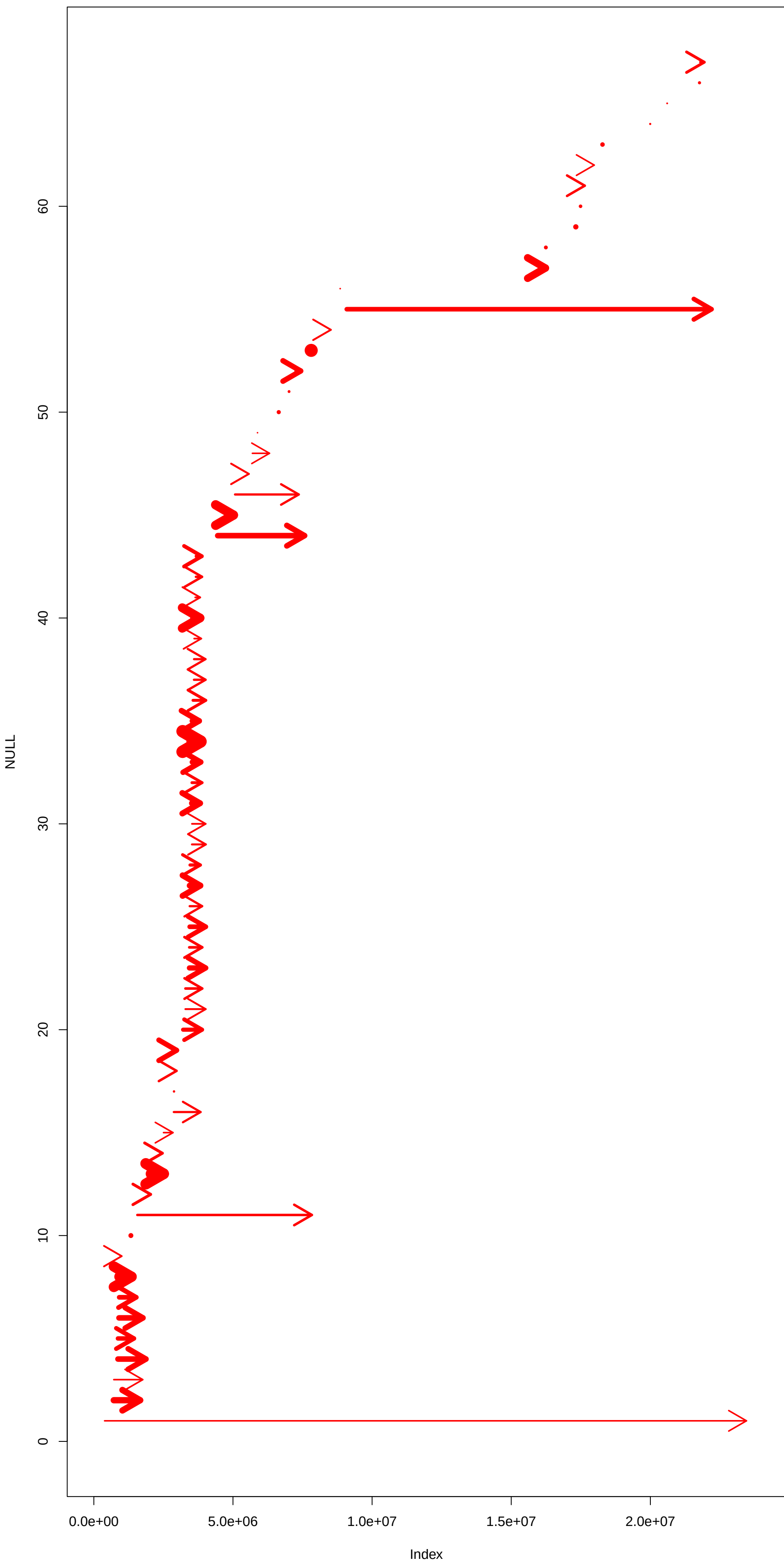
NC_044069.1
