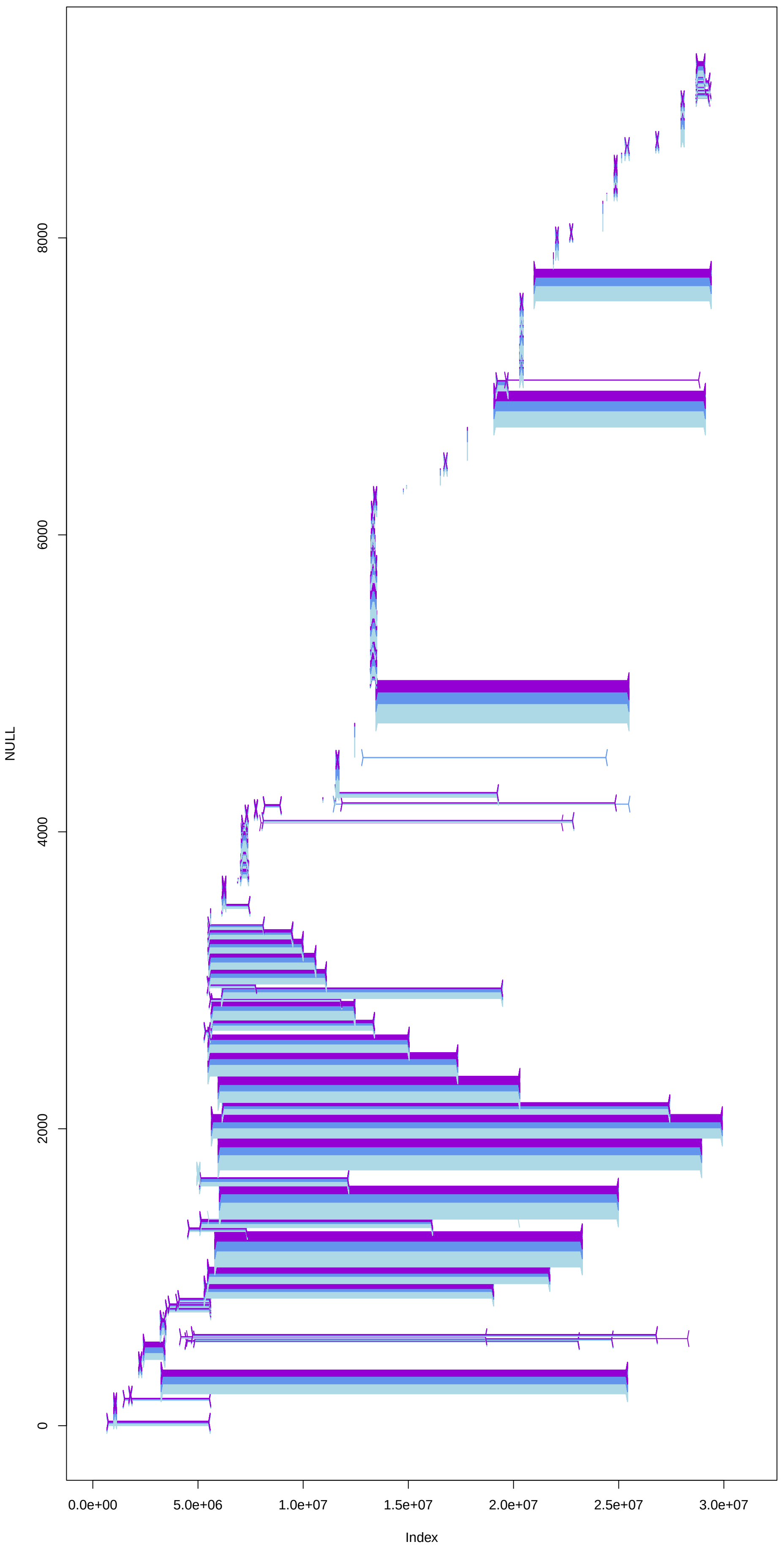
NC_044048.1
