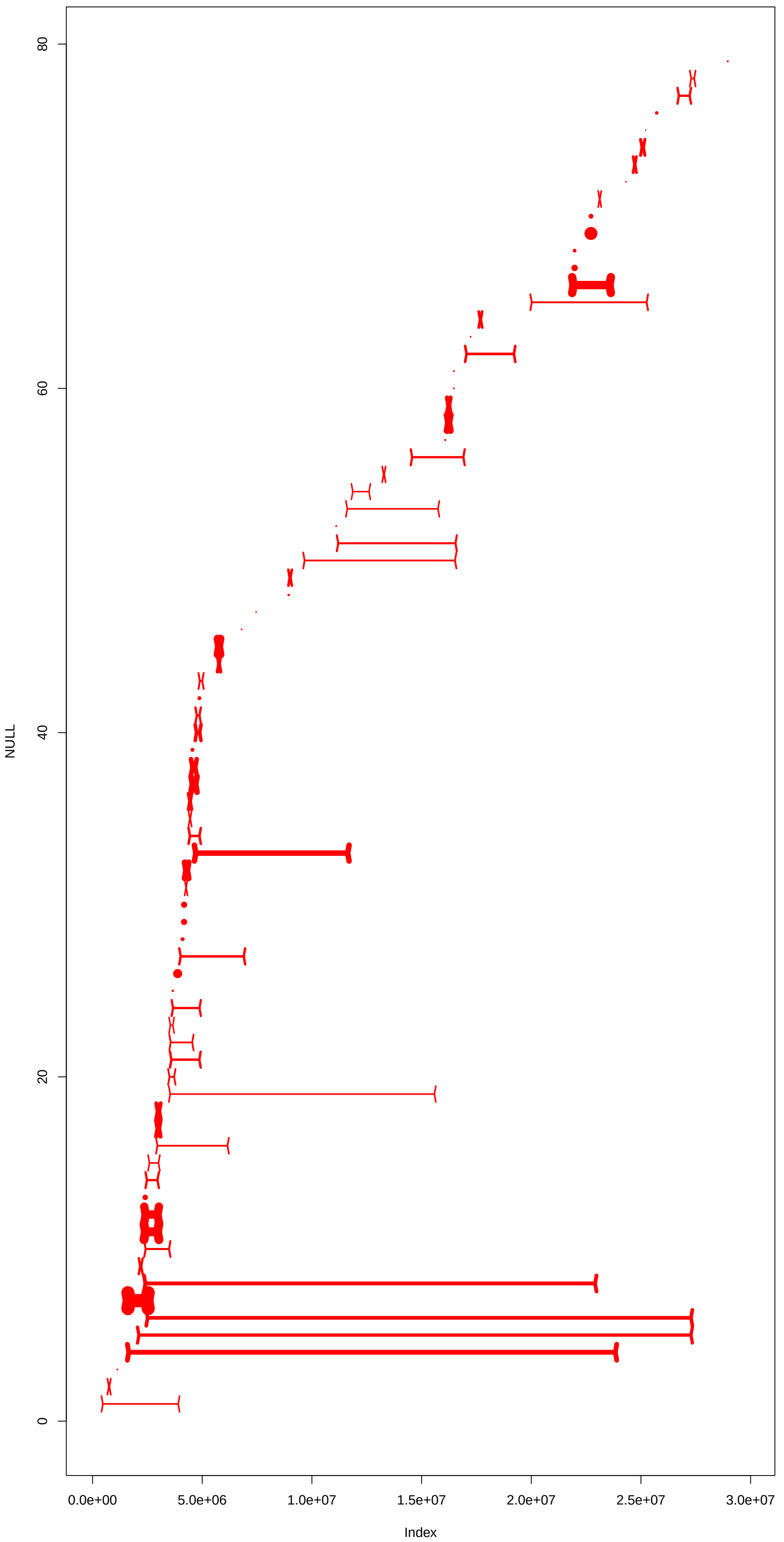
NC_044055.1 pass1
