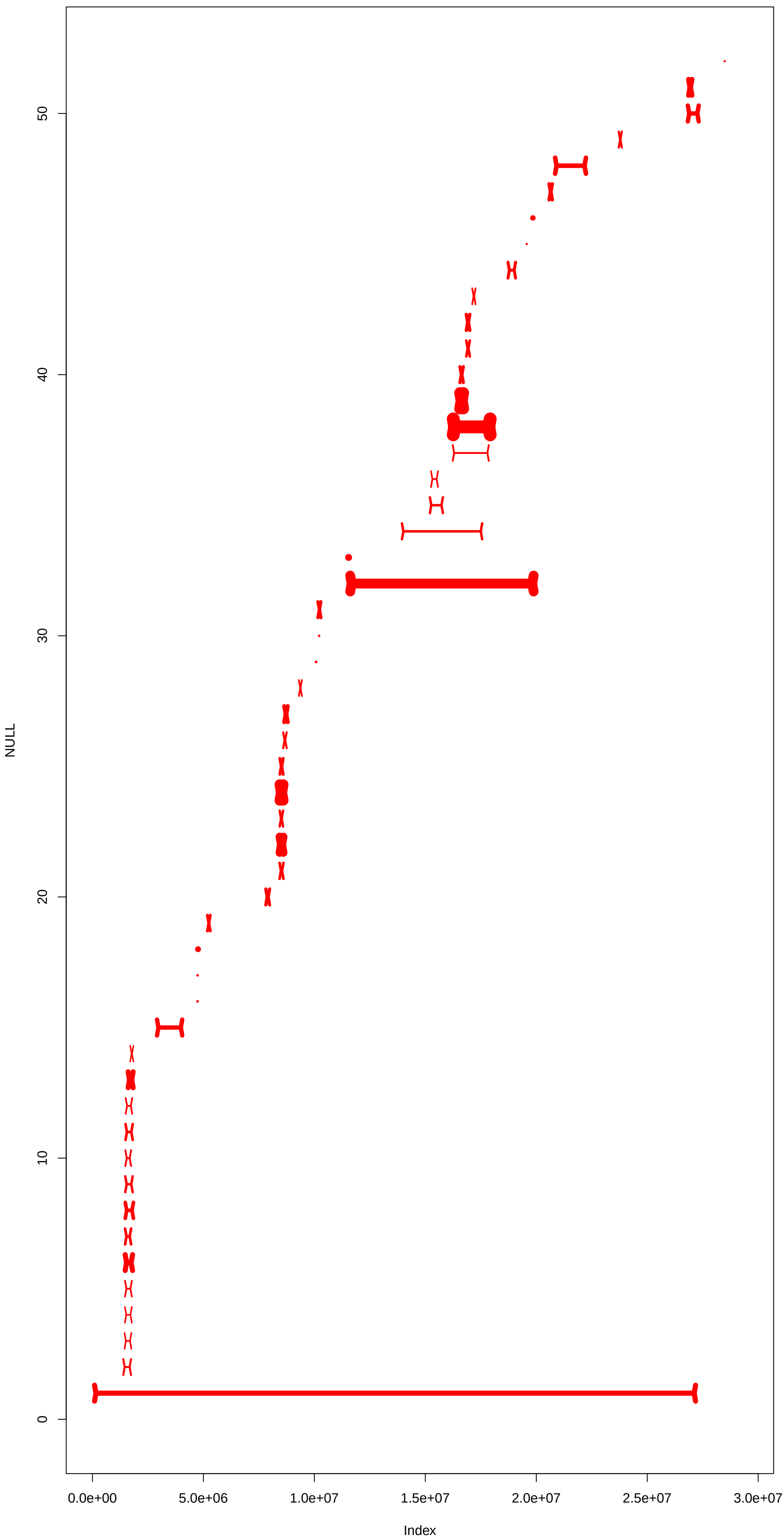
NC_044061.1 pass1
