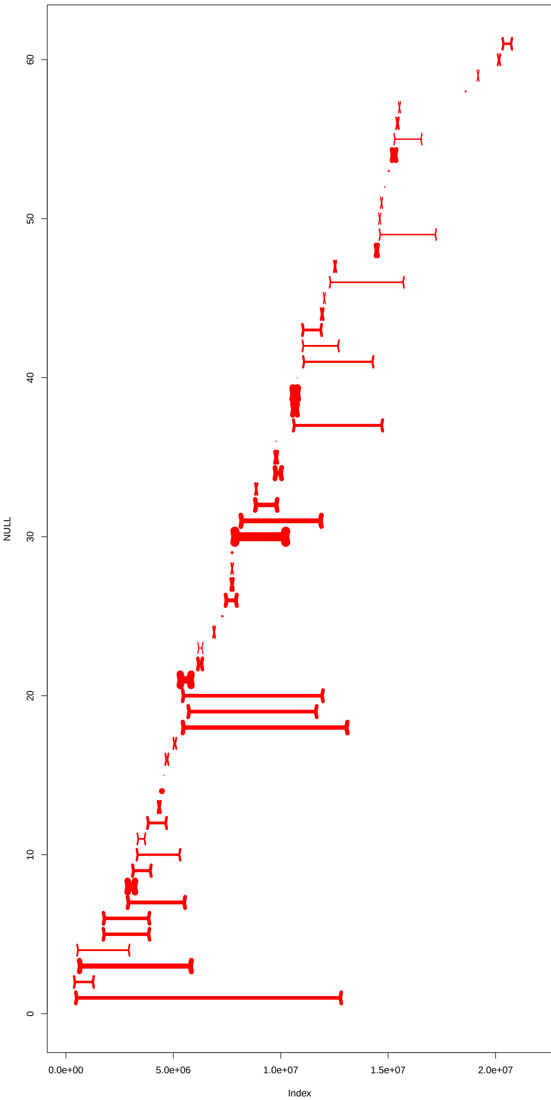
NC_044064.1 pass1
