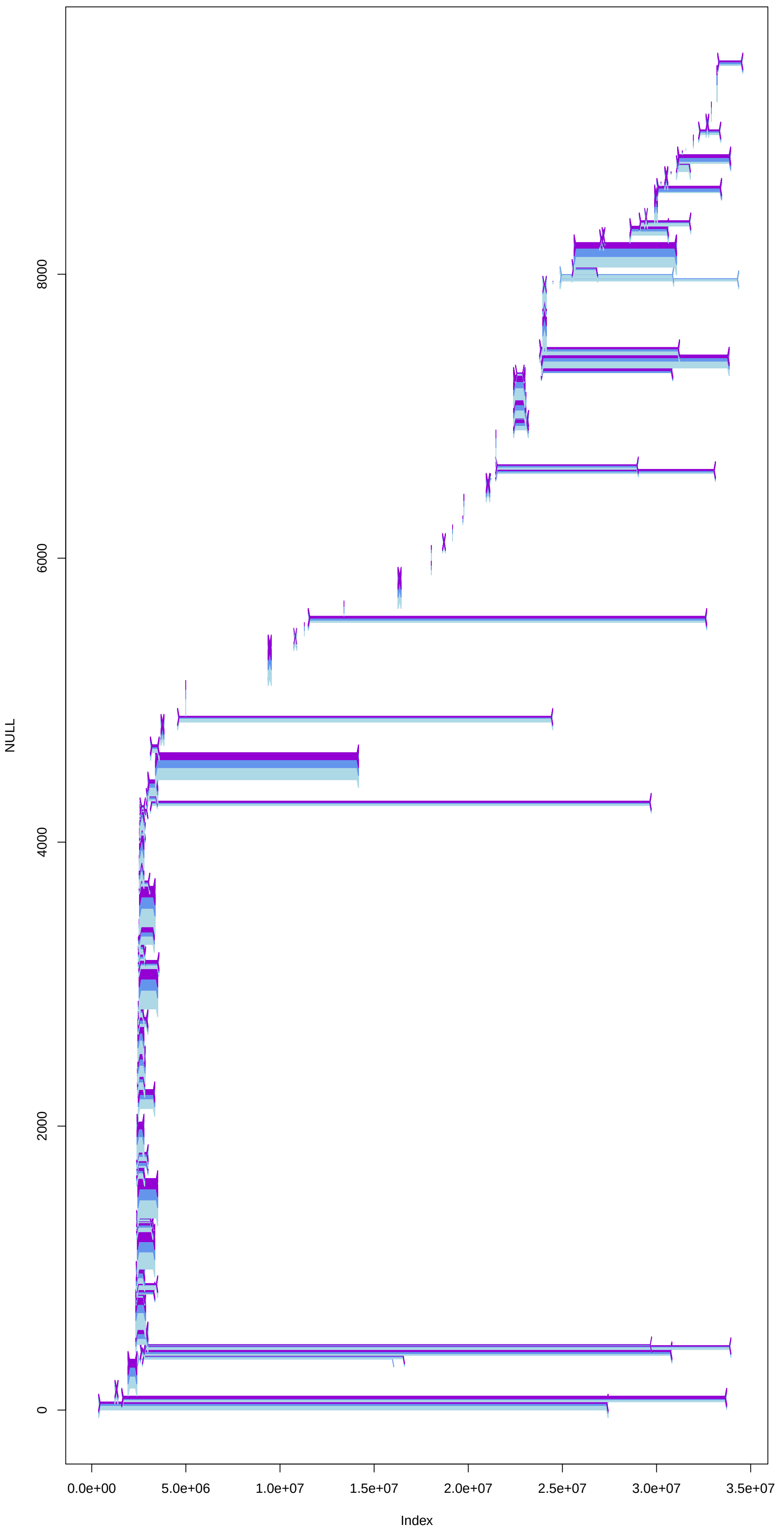
NC_044063.1
