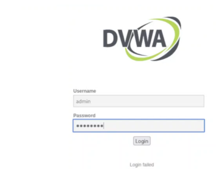
Рис. 2.4: Авторизация
