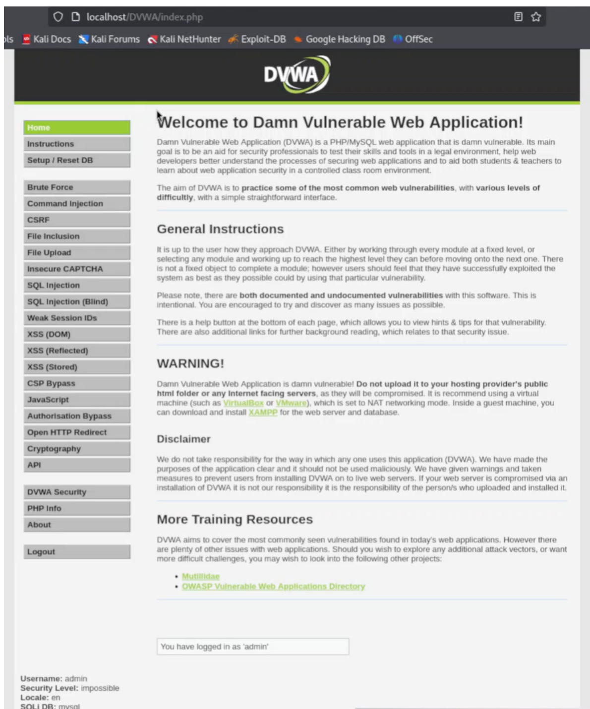
Рис. 2.5: Настроенный сайт
