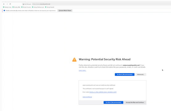
Рис. 6: Предупреждение
