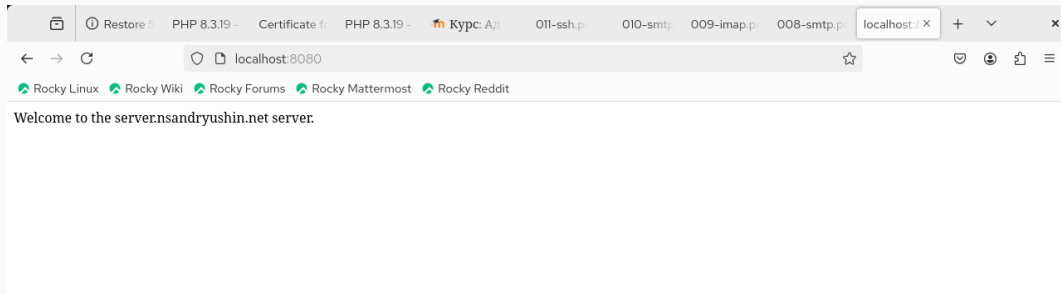
Рис. 27: Результат переадресации
