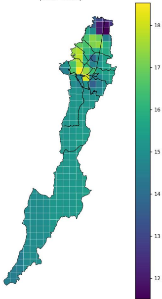
NO2 interpolado promedio (2020-2024)
