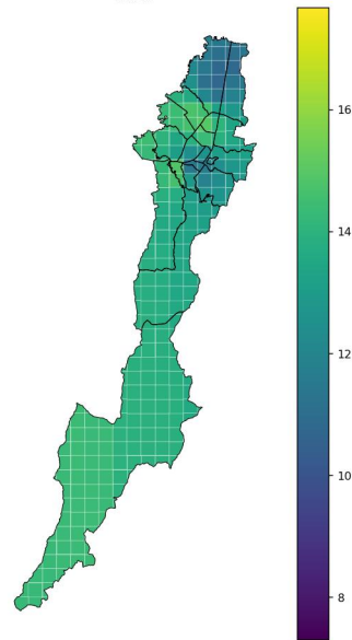
O3 promedio 2024
