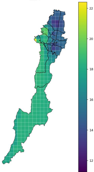
PM2.5 promedio 2024
