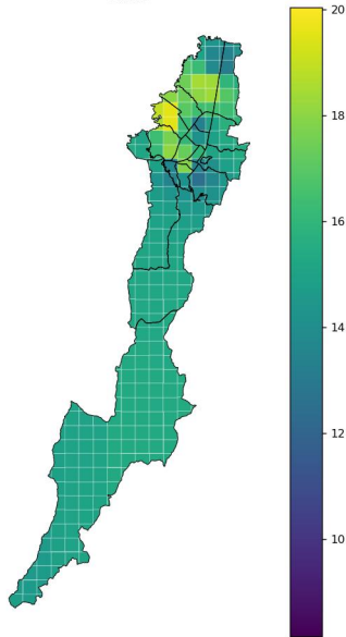
NO2 promedio 2024
