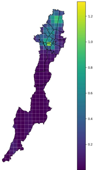
Gradiente NO2 2023
