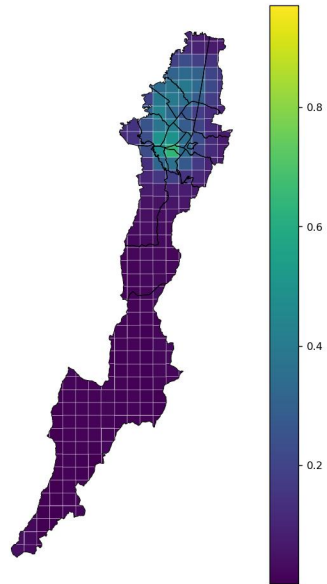
Gradiente O3 2023
