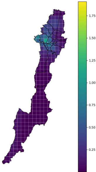
Gradiente PM2.5 2023
