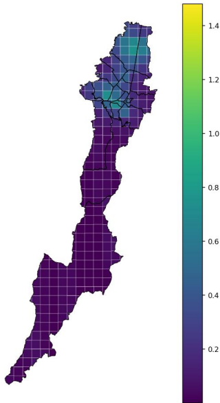
Proxy advectivo NO2 2021
