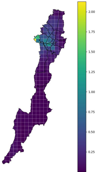
Proxy advectivo PM2.5 2021
