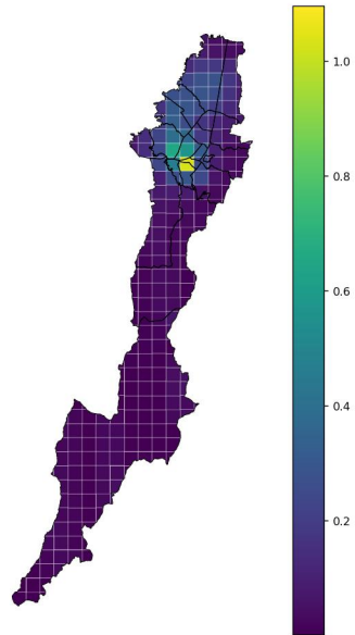
Proxy advectivo O3 2021
